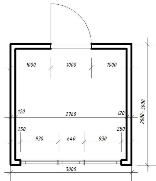
ПЛАН ТИМЧАСОВОЇ СПОРУДИ
