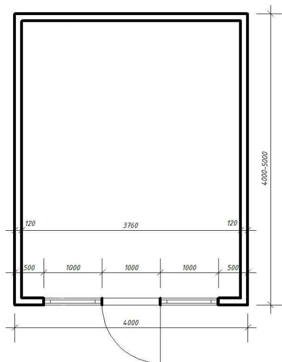
ПЛАН ТИМЧАСОВОЇ СПОРУДИ
